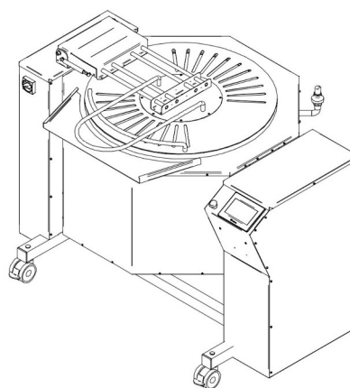
VISTA ISOMÉTRICA
