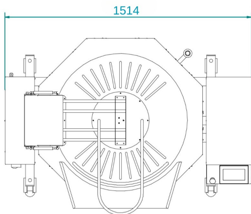
VISTA PLANTA
